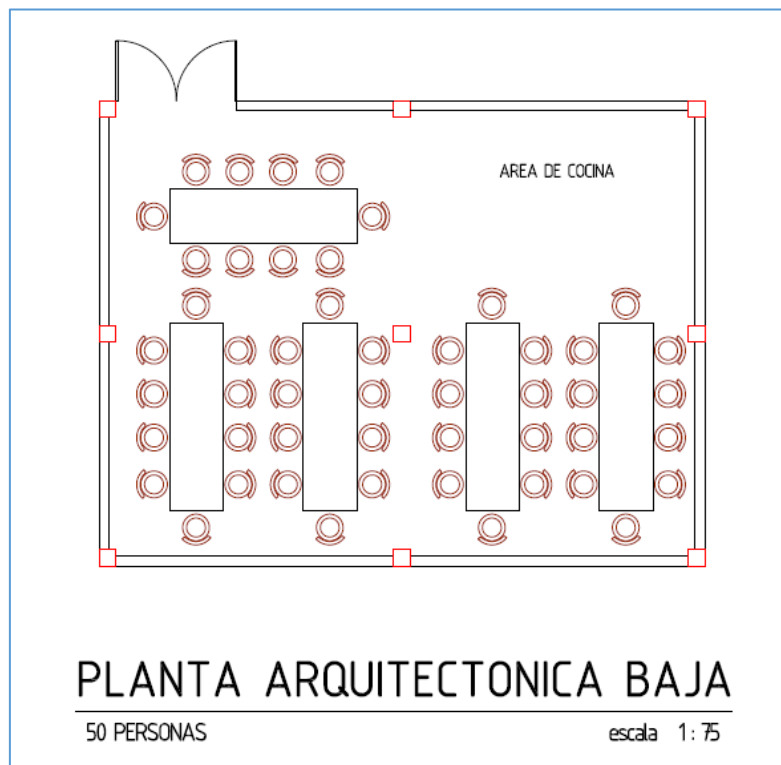
Figura 1: Distribución de los espacios (Planta Baja)
