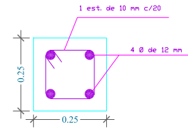
DETALLE DE COLUMNA
