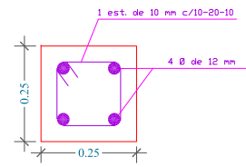
DETALLE DE CADENA
