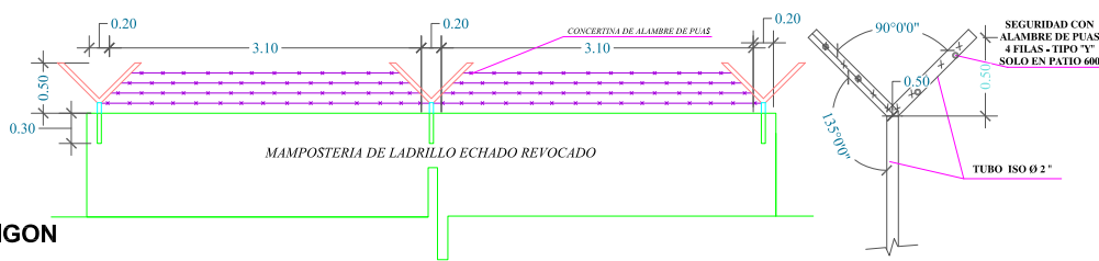
DETALLE DE CONCERTINA ALAMBRE DE PUA
