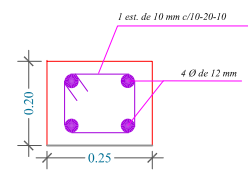
DETALLE DE VIGA HORMIGON ARMADO
