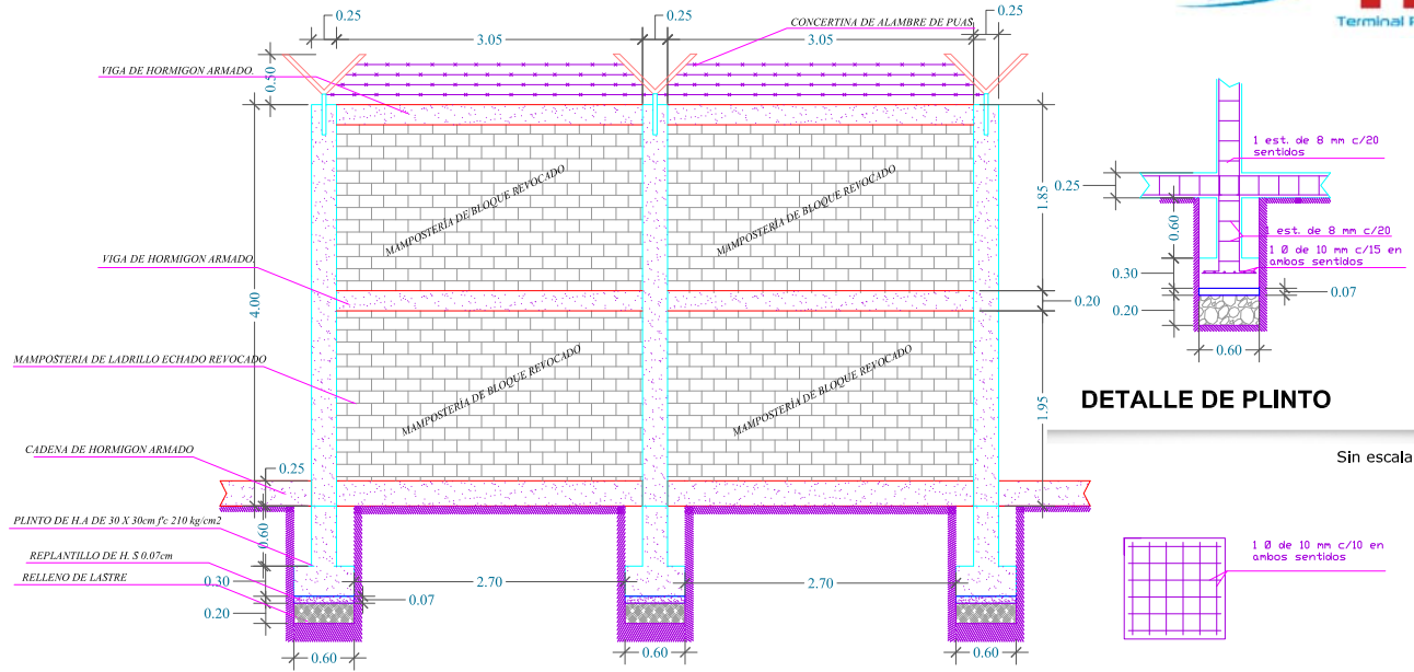
DETALLE DE ARMADURA
